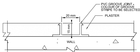
TYP. GROOVE JOINT 1:1
